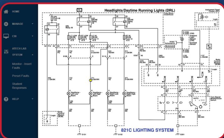
Wiring schematics
